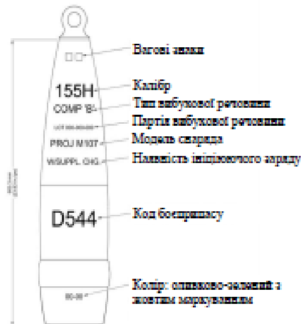
Рисунок Д1.1 – Маркування 155-мм артилерійських снарядів
